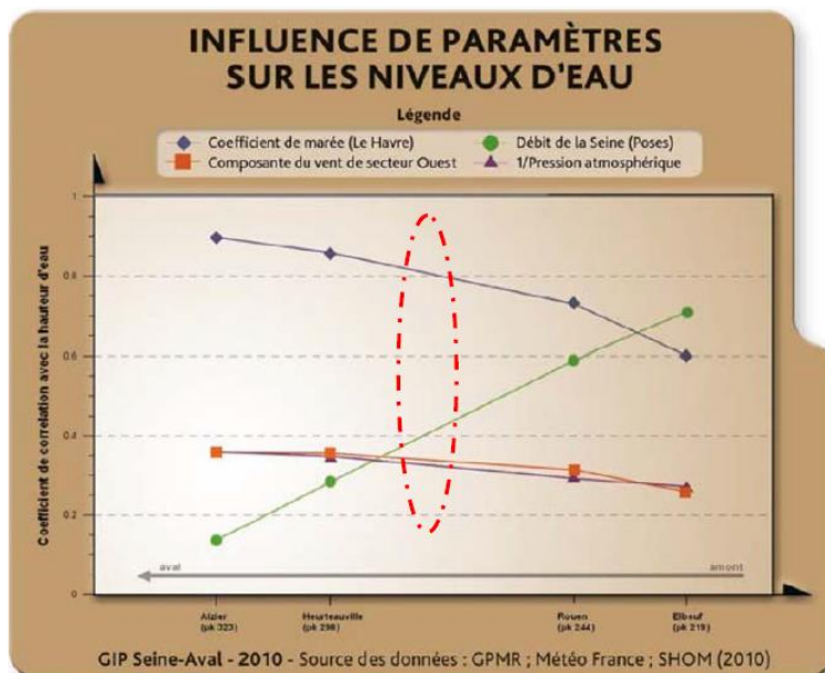
Figure 84 : Influence des 4 paramètres hydro-climatiques sur le niveau d'eau de la Seine au droit de la zone d'étude (source SGEP)
