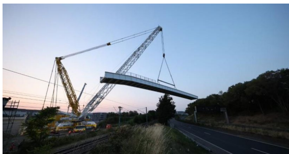
Opération de grutage du tablier de la passerelle qui relie le quartier de la Piscine au centre-ville du Petit Quevilly au-dessus la Sud 3 et la voie de chemin de fer
