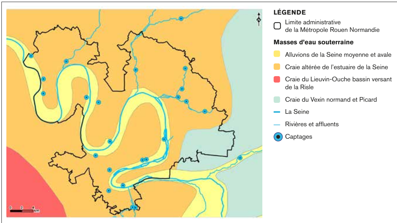
FIGURE 2 : Captages exploités pour l'alimentation en eau potable (AEP) de la Métropole
