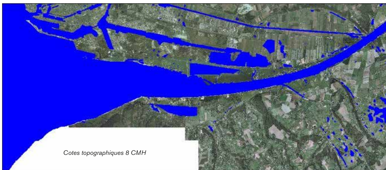
FIGURE 9.a : Modélisation du niveau moyen de pleine mer en vive-eau (cote 8 CMH) de l'embouchure de la Seine – Sources : IGN, PAR, PAH, MDE
