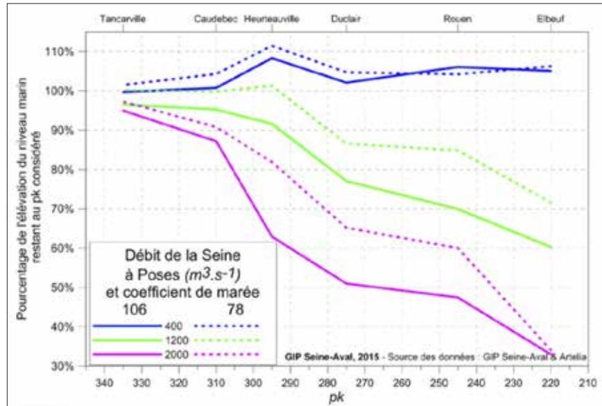
FIGURE 8 : Impact de l'élévation du niveau marin sur les niveaux de pleine mer avec des coefficients de 78 et 106 calculés pour des débits différents de la Seine à Poses. – Sources : Lemoine, 2015.
